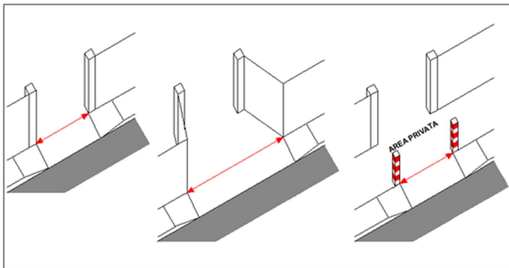
Esempi di misurazione della larghezza dell'accesso carrabile
